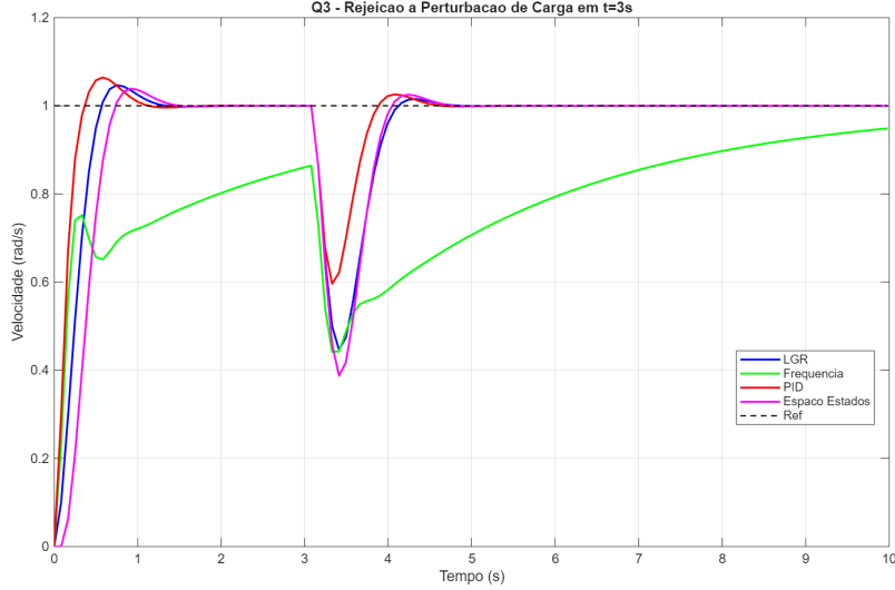
Figura 8: Resposta à perturbação de carga T_d = degrau unitário.
